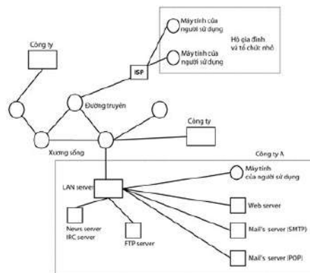
Hình 16.1. Mạng Internet
